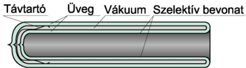
Kettősfalú, "Sydney" típusú vákuumcső
