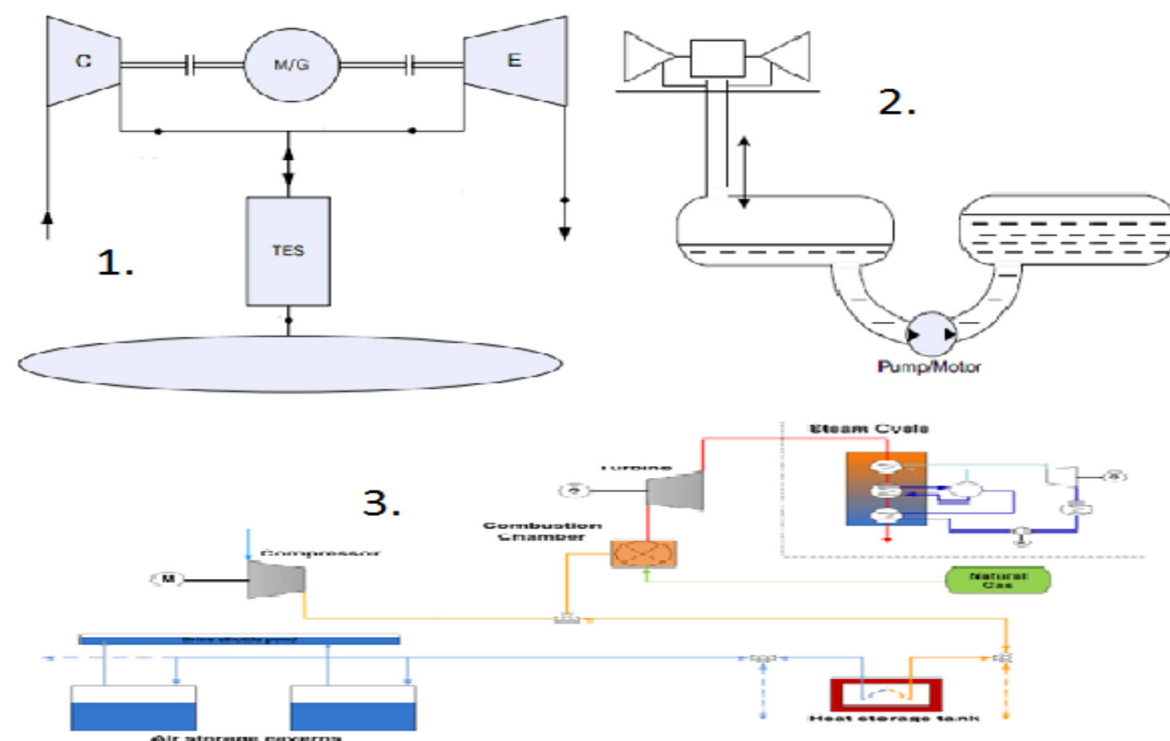
1. Adiabatikus CAES; 2. CAES és SZET kombinációja; 3. ISACOAST-CC
