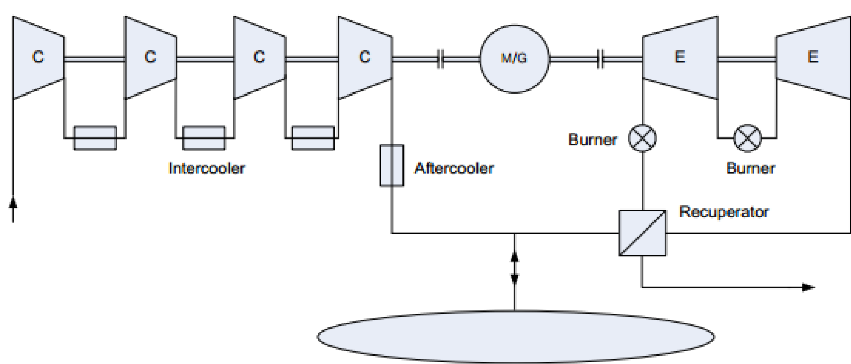
A McIntosh-i erőmű kapcsolása
